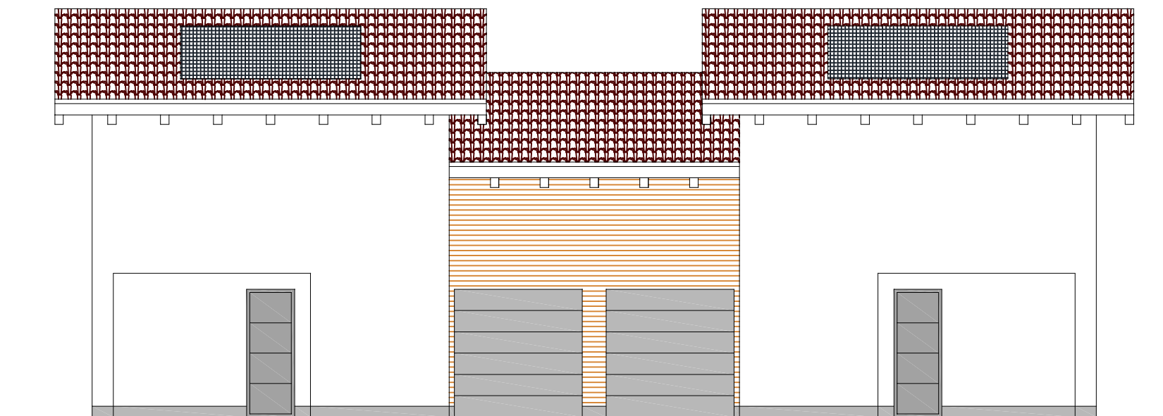
prospetto ovest
